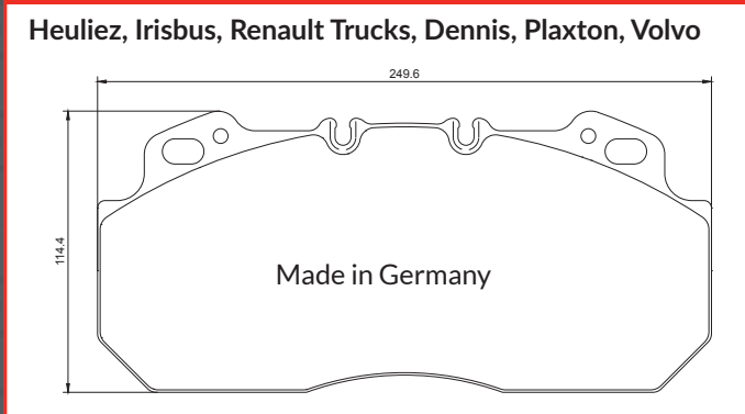
CVP112K (29279) Wabco Maxx 22
