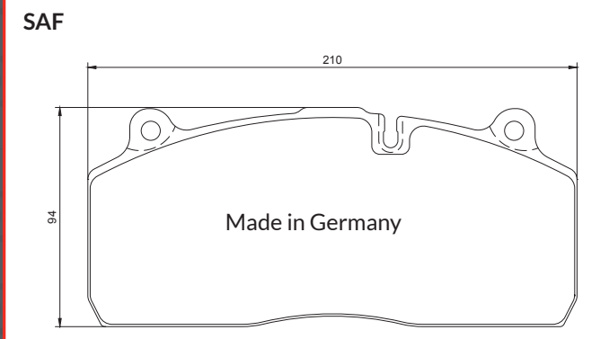
CVP092K (29306) Knorr SN 6
