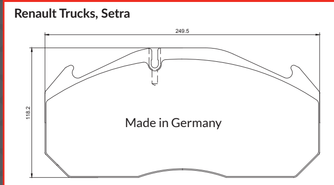
CVP090K (29313) Wabco PAN 19-1
