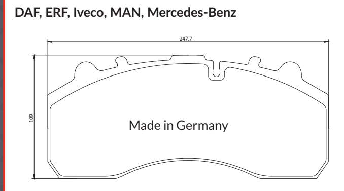
CVP038K (29136) Meritor B-DUCO
