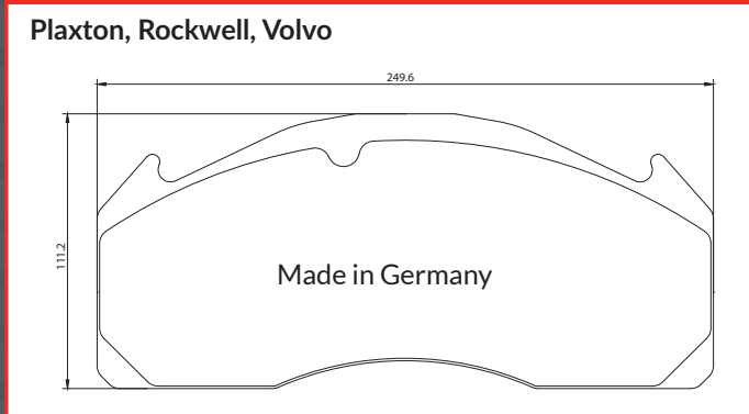
CVP101K (29174) Meritor ELSA 225-3
